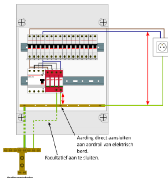
Figuur 14: correcte aansluiting van de aarding
