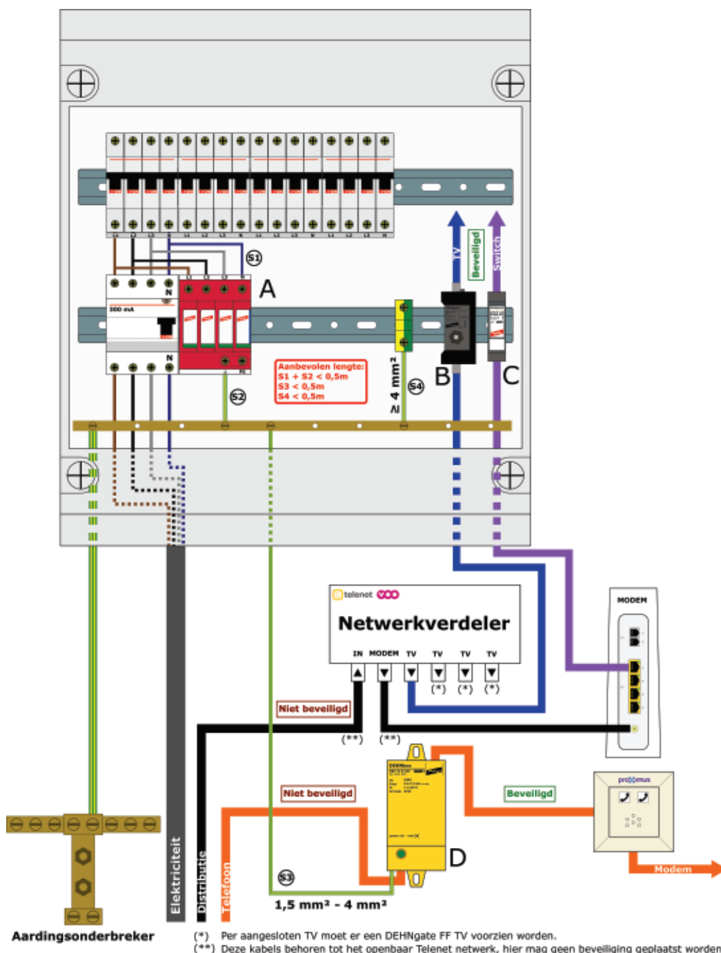
Figuur 10: algemeen principe overspanningsbeveiliging voor een woning
