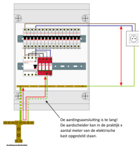
Figuur 13: foutieve aansluiting van de aarding
