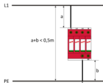
Figuur 11: installatierichtlijn voor overspanningsbeveiligingen
